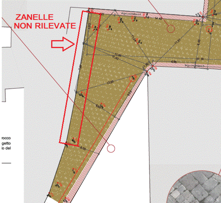
STRALCIO TAVOLA RILIEVO DELLO STATO DI FATTO
