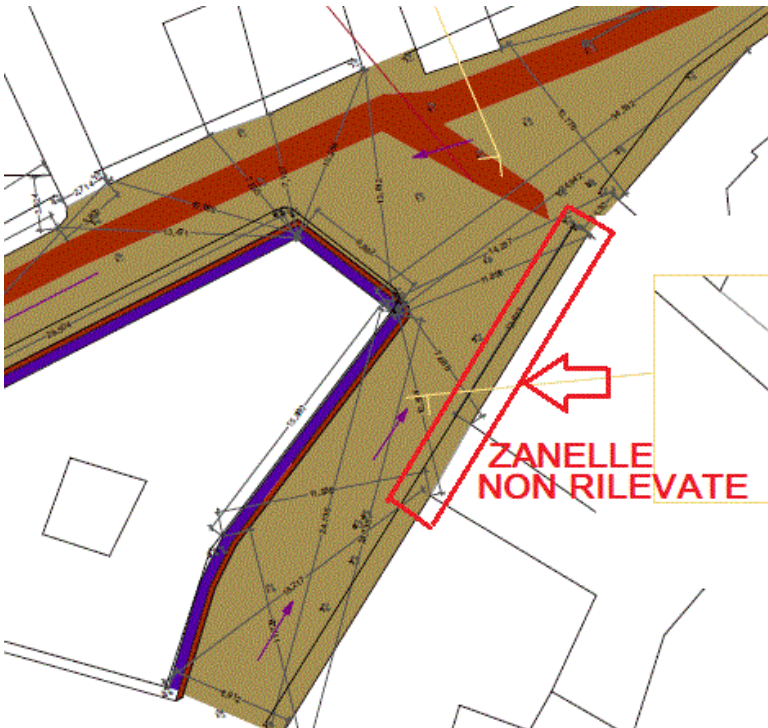
STRALCIO TAVOLA RILIEVO DELLO STATO DI FATTO
